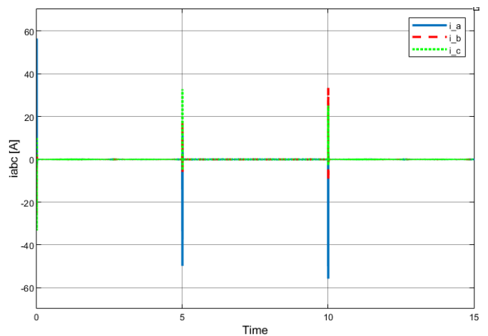
Figura 46: Corrientes i_{abc}(t)
