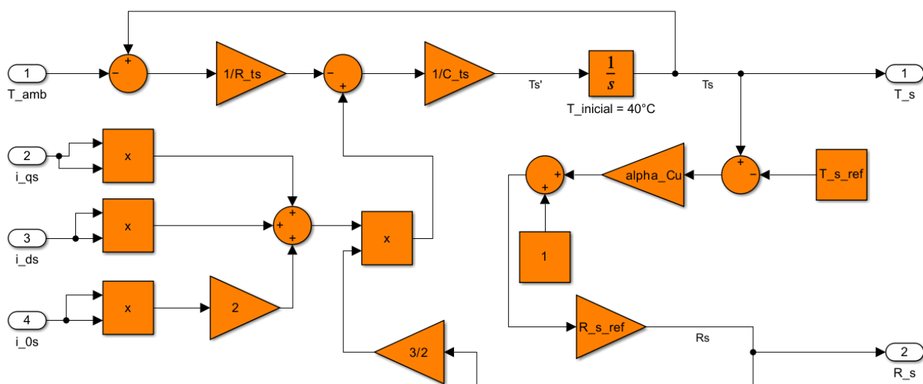
Figura 5: Subsistema térmico
